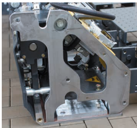
Semplicità stupefacente: sistema di riscaldamento con monitoraggio dei circuiti di riscaldamento.
