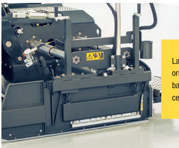
Paratie laterali riscaldabili.
